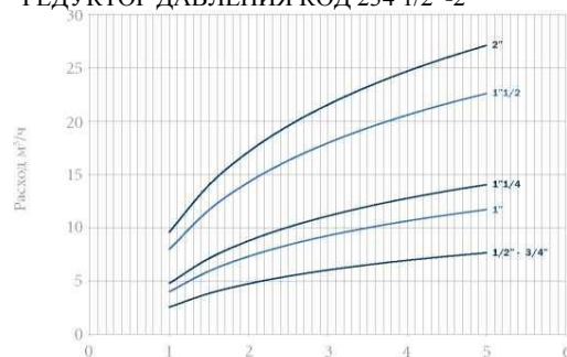
РЕДУКТОР ДАВЛЕНИЯ КОД 234 1/2"-2"
